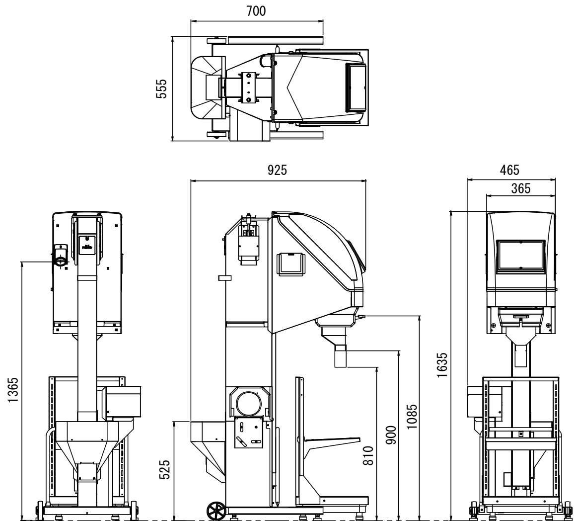
図 6 機体寸法図
