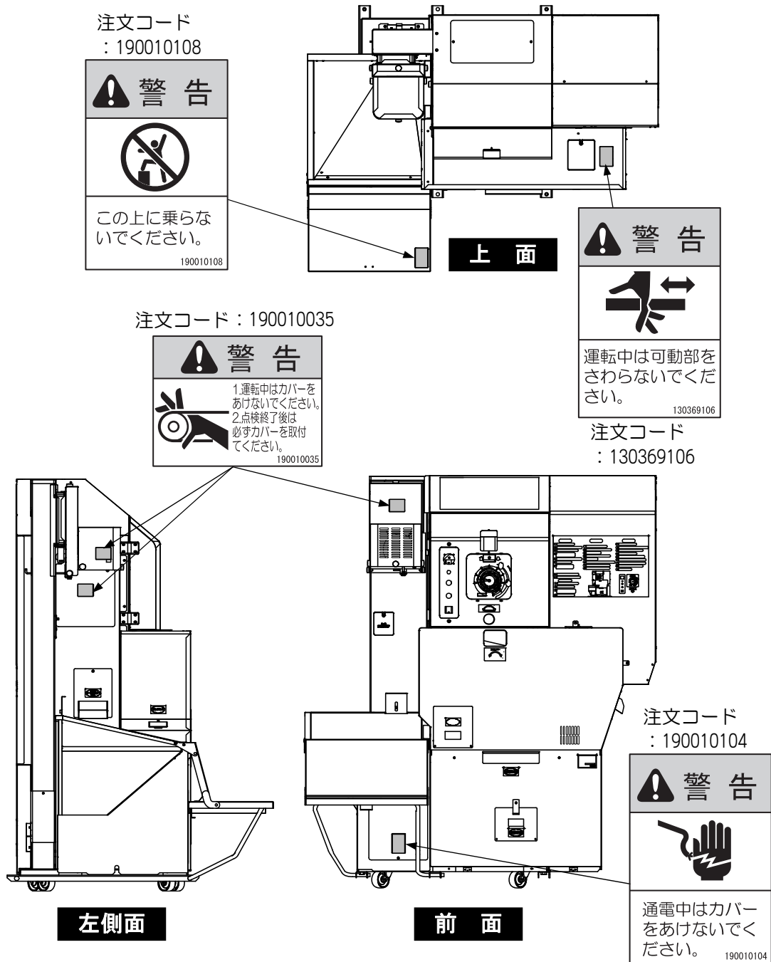
図1 標示ラベル貼付位置(1)
