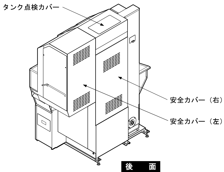
図 4 機械全体図 (2)
