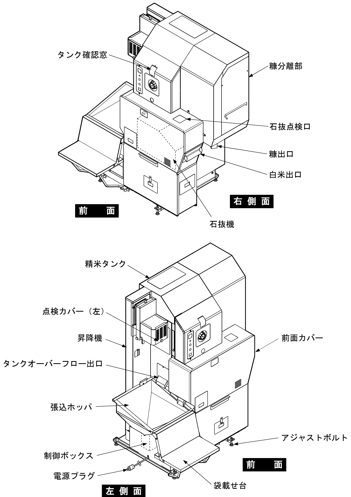
図 3 機械全体図 (1)
