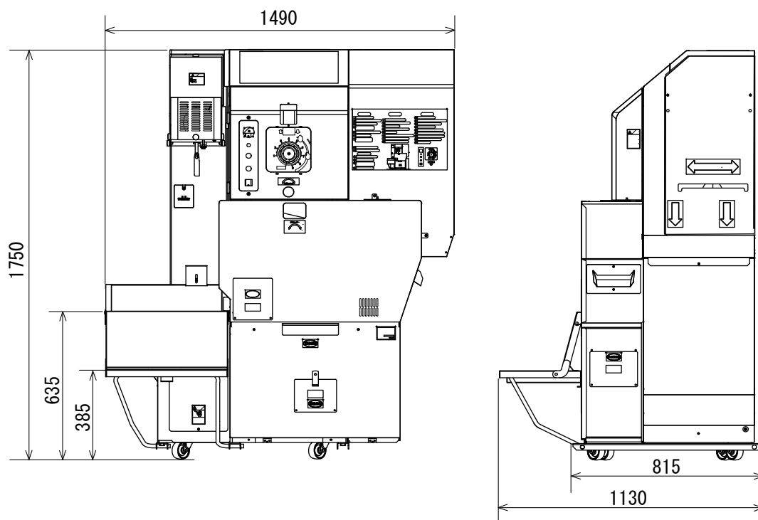
図 8 寸法図
