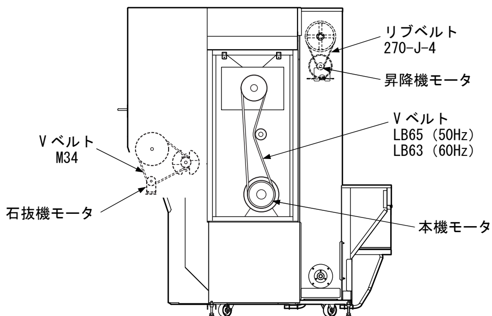
図 9 V ベルトの掛け方
