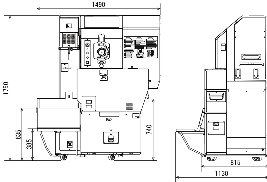
図 8 寸法図
