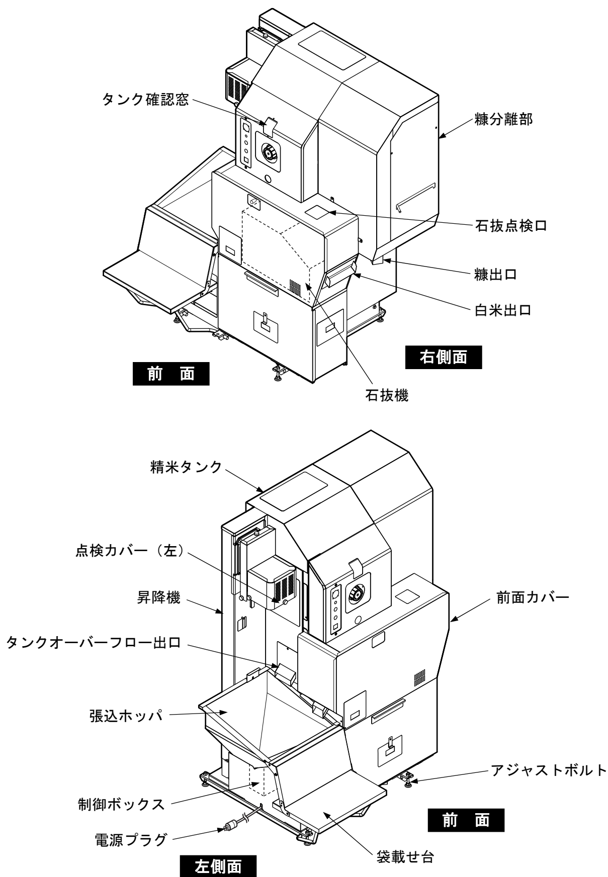
図 3 機械全体図 (1)
