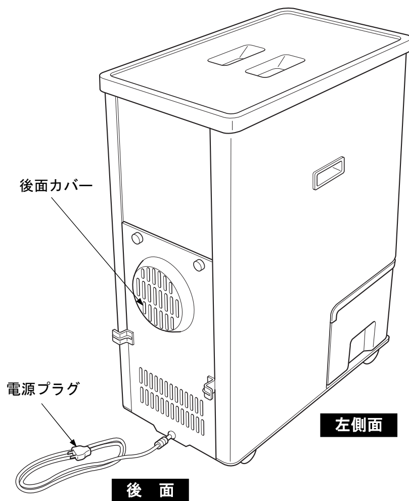
図 3 機械全体図 (2)
