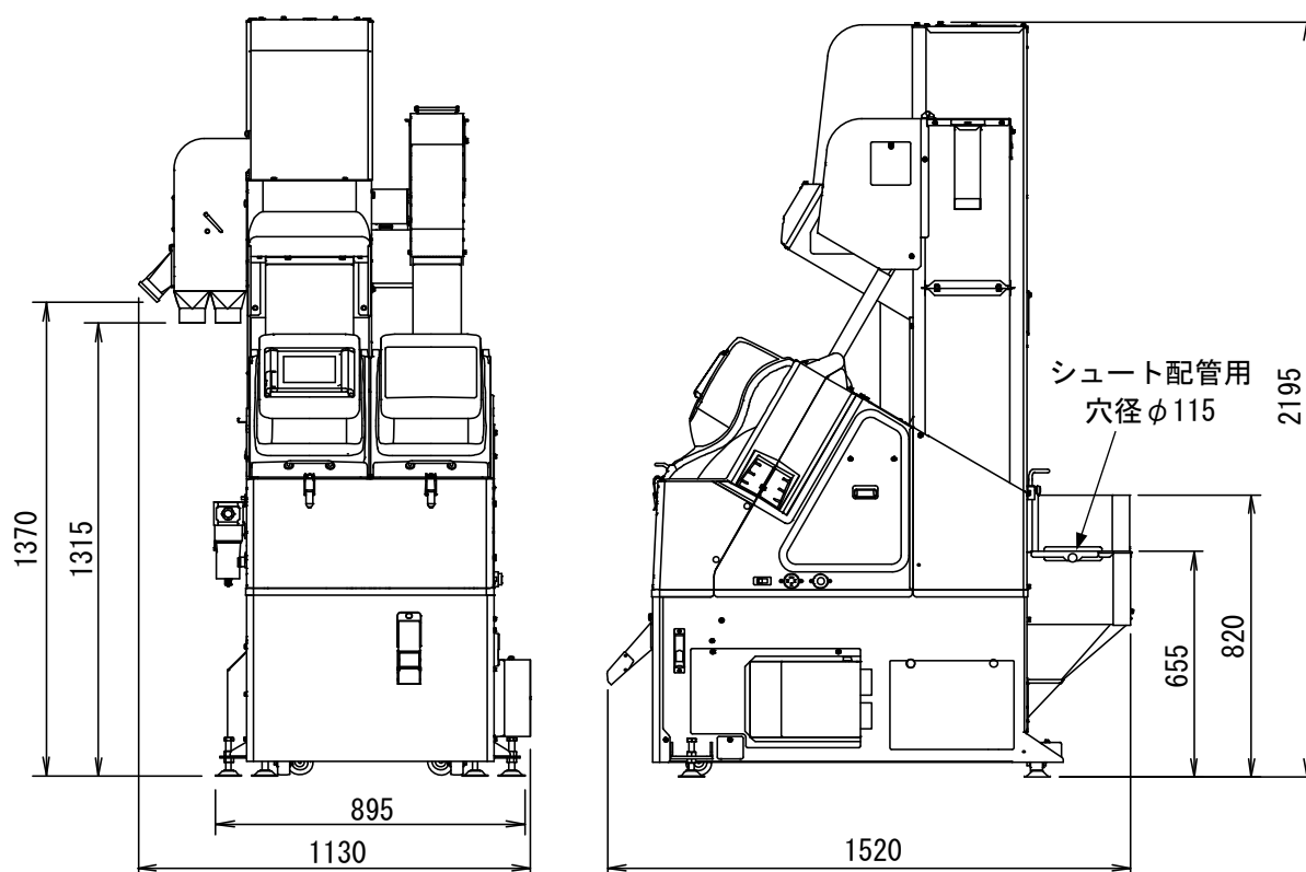
図 8 機体寸法
