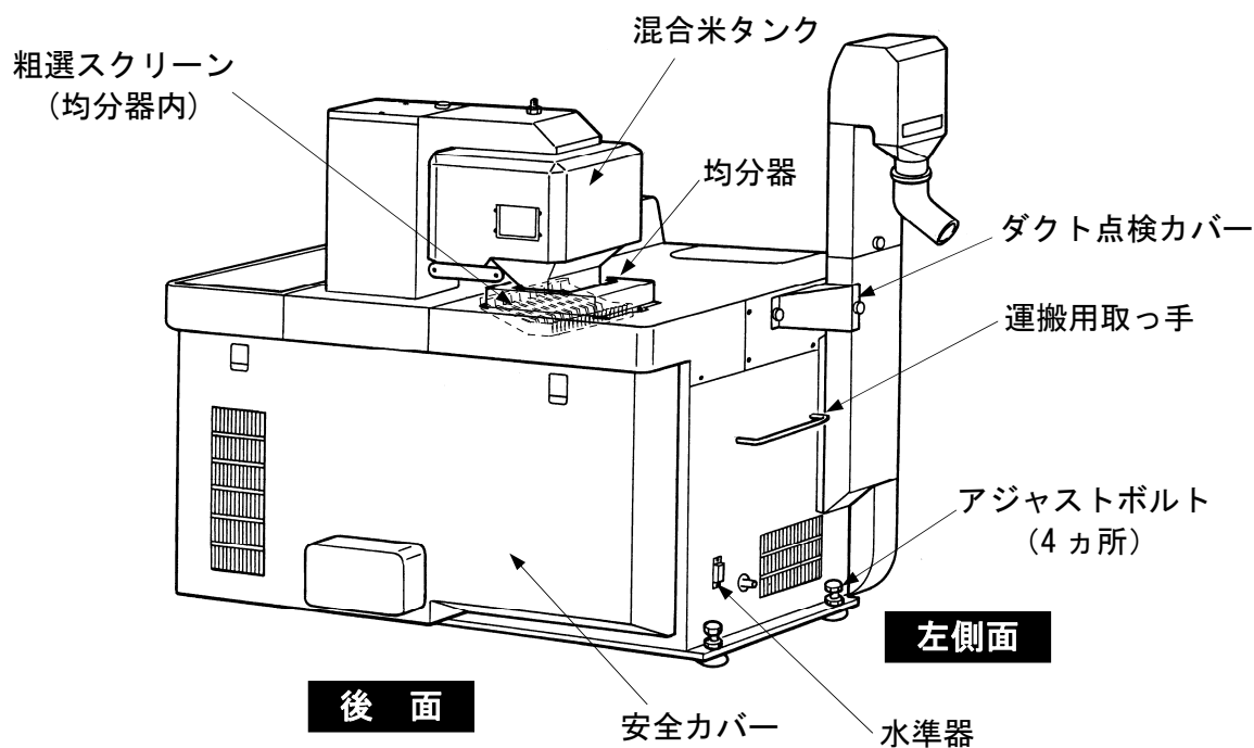
図 4 機械全体図 (2)
