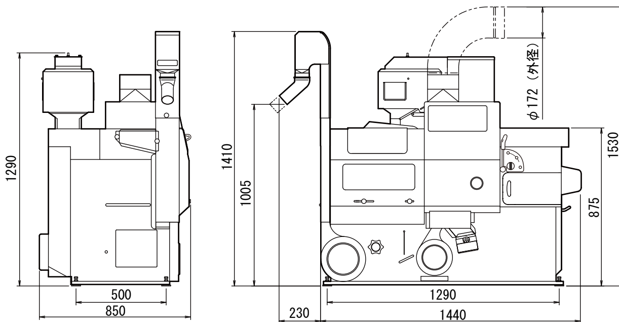
図 8 機体寸法
