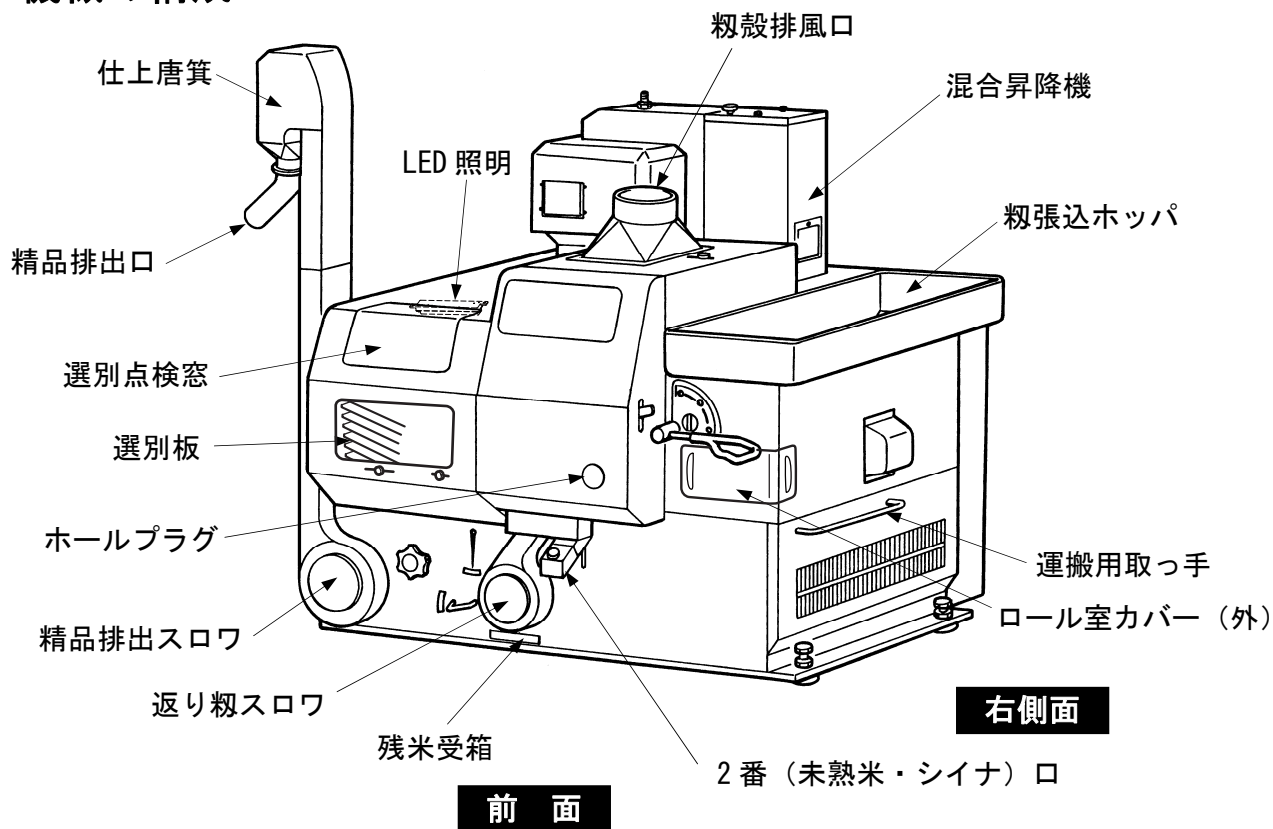
図 3 機械全体図 (1)
