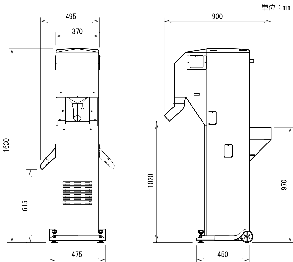
図 5 機械寸法
