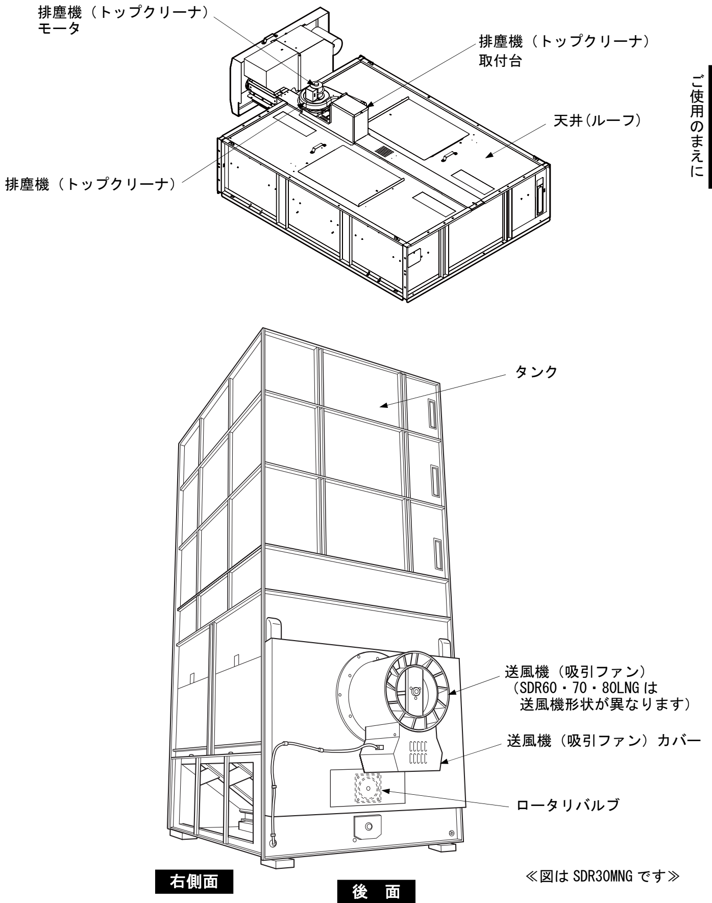
図 4 機械全体図（2）
