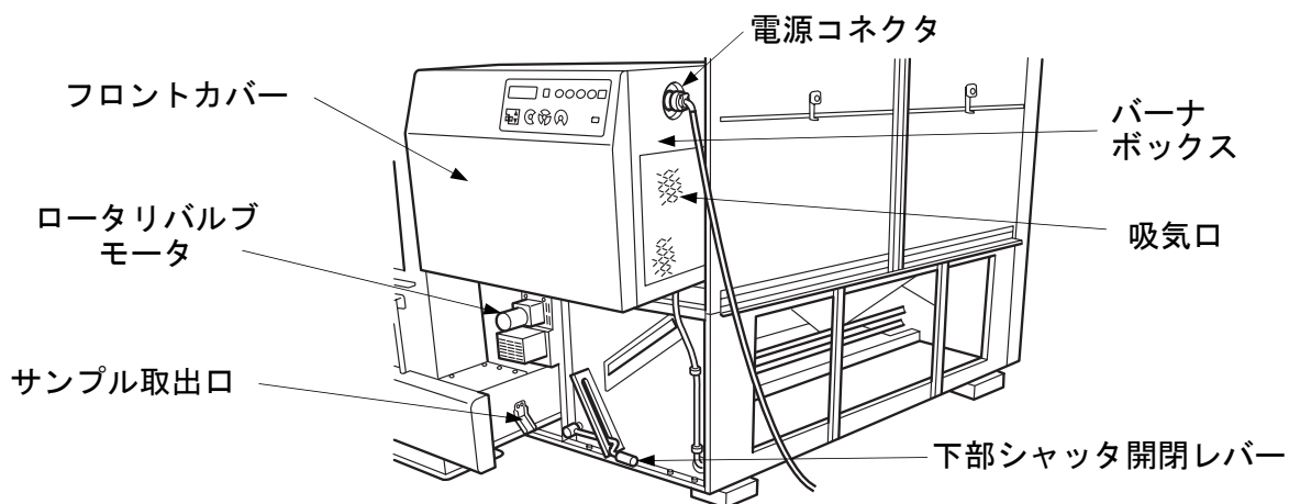
図 3 機械全体図 (1)
