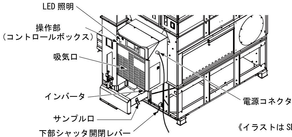
図 3 機械全体図 (1)
