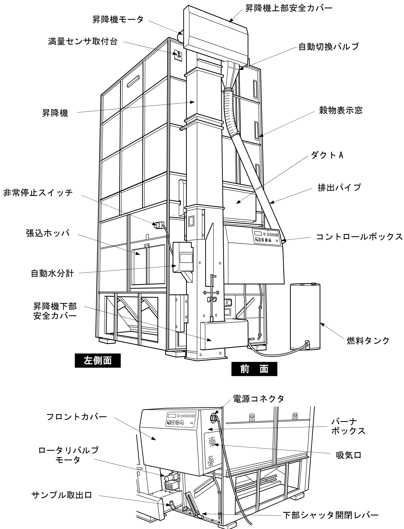
図 3 機械全体図 (1)
