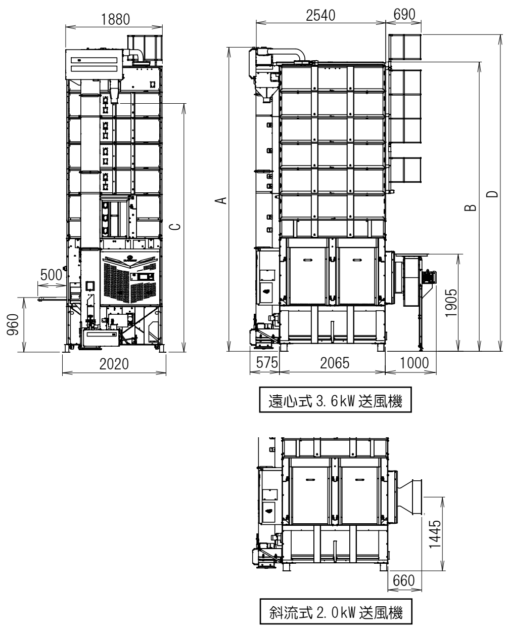
図 5 機体寸法
