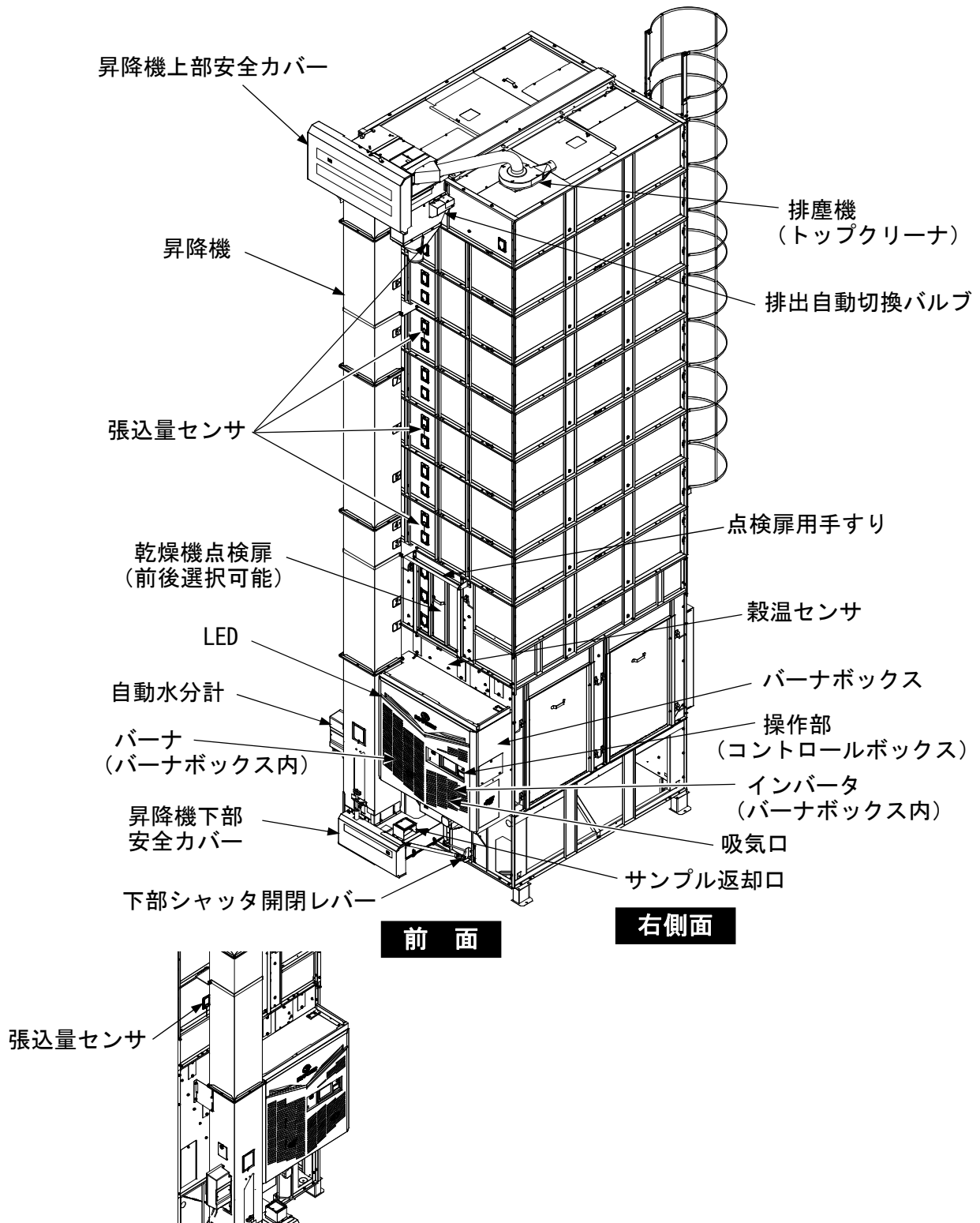
図 3 機械全体図 (1)
