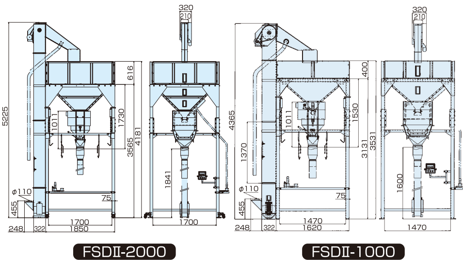
寸法 (mm) FSD II - 1000/2000
